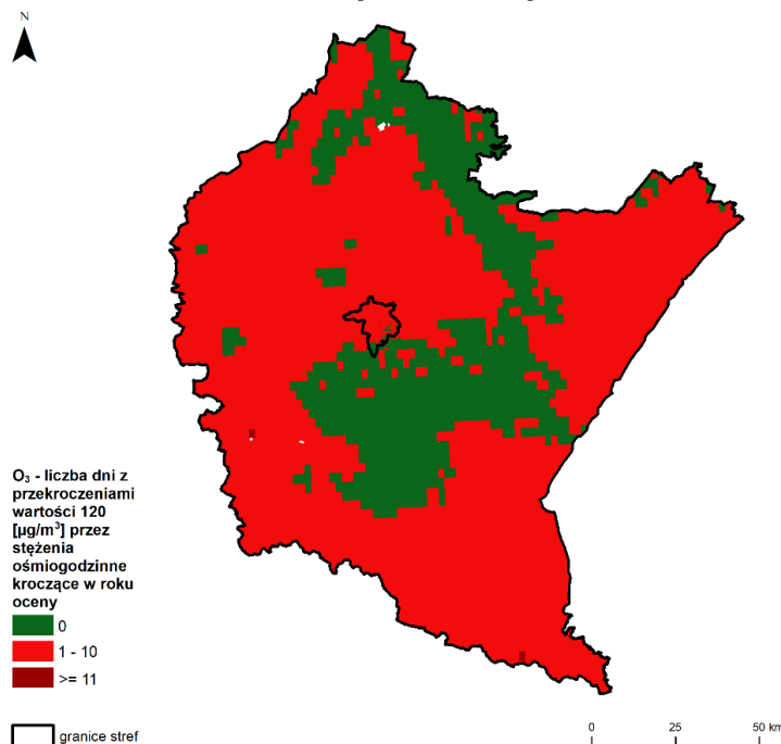
Rysunek 16 Rozkład przestrzenny liczby dni z przekroczeniem poziomu celu długoterminowego O_3 na obszarze woj. podkarpackiego w 2023 r., opracowany z wykorzystaniem metody szacowania w oparciu o wyniki modelowania jakości powietrza dla roku 2022 wykonanego przez IOŚ-PIB [źródło: GIOŚ, IOŚ-PIB]
