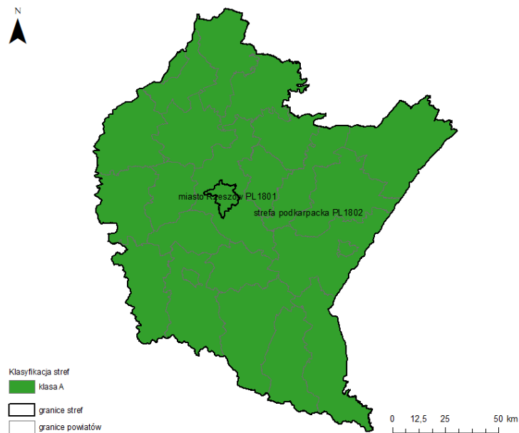
Rysunek 12 Klasyfikacja stref w województwie podkarpackim dla benzenu dla średniorocznego czasu uśredniania, z uwzględnieniem kryteriów określonych w celu ochrony zdrowia – 2023 r.
