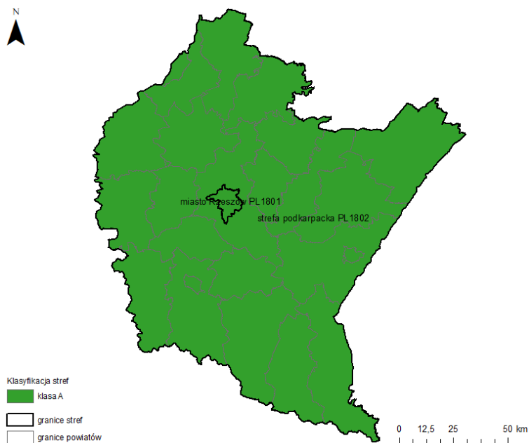
Rysunek 10 Klasyfikacja stref w woj. podkarpackim dla dwutlenku siarki dla czasu uśredniania – 24 godz., z uwzględnieniem kryteriów określonych w celu ochrony zdrowia – 2023 r. [źródło: GIOŚ]
