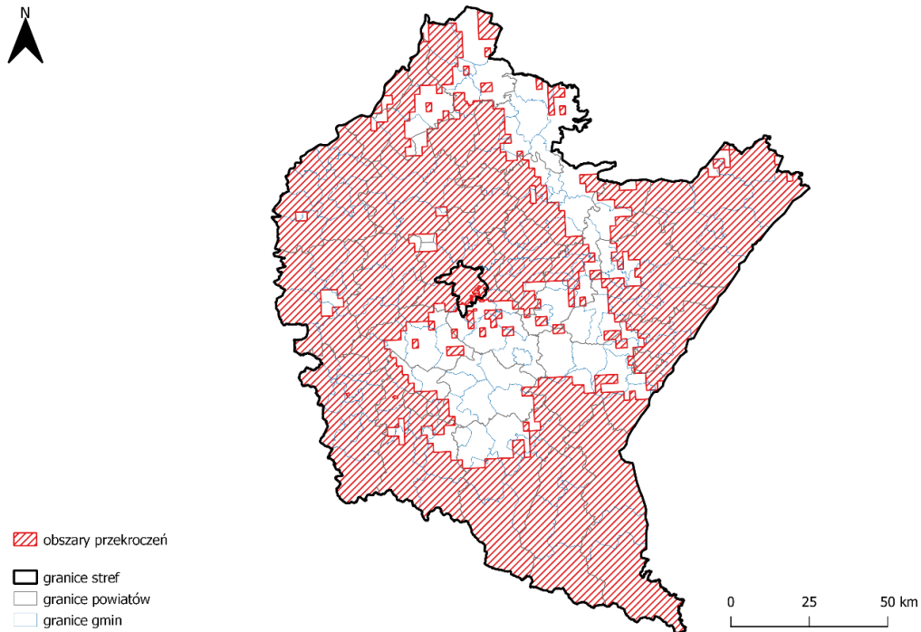
Rysunek 17 Zasięg obszarów przekroczeń poziomu celu długoterminowego ozonu dla 8-godz. stężenia O_3 ze względu na ochronę zdrowia w województwie podkarpackim w 2023 r. [źródło: GIOŚ]
