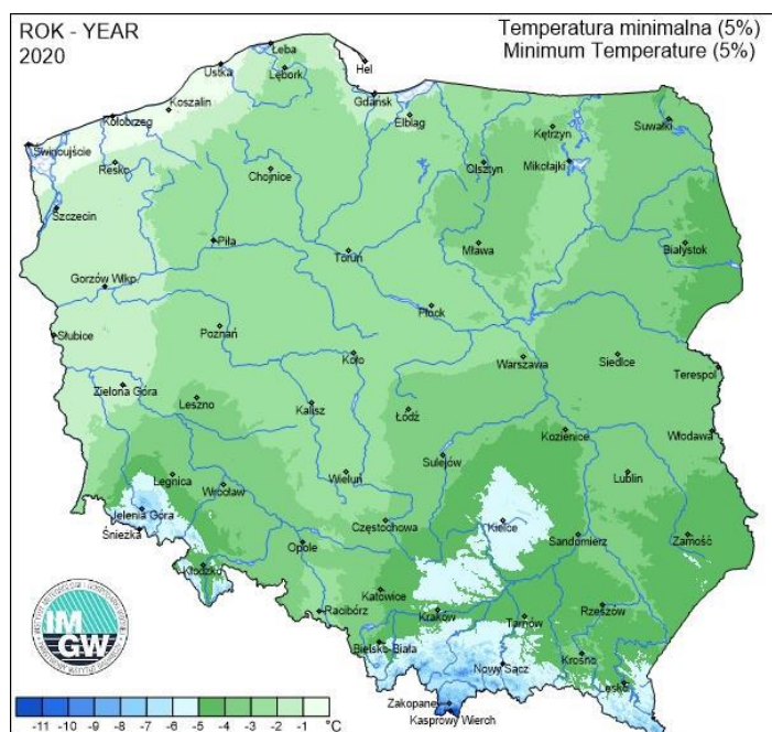
Rysunek 8 Przestrzenny rozkład wartości temperatury powietrza w Polsce w 2020 r. – temperatura minimalna. Źródło: Roczna ocena jakości powietrza w województwie podkarpackim
