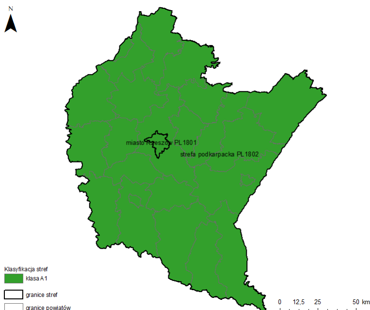
Rysunek 14 Klasyfikacja stref w woj. podkarpackim dla pyłu PM 2,5 , dla średniorocznego czasu uśredniania-faza II, z uwzględnieniem kryteriów określonych w celu ochrony zdrowia – 2023 r. [źródło: GIOŚ]
