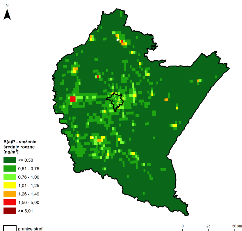
Rysunek 20 Rozkład przestrzenny wartości stężenia średniego rocznego B(a)P w województwie podkarpackim w 2023 r., opracowany z wykorzystaniem metody szacowania w oparciu o wyniki modelowania jakości powietrza dla roku 2023 wykonanego przez IOŚ-PIB [źródło: GIOŚ, IOŚ-PIB]
