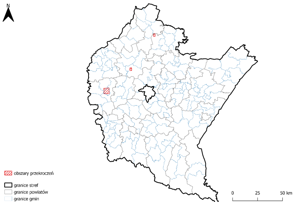
Rysunek 19 Zasięg obszarów przekroczeń poziomu docelowego benzo(a)pirenu określonego ze względu na ochronę zdrowia w województwie podkarpackim w 2023 roku (źródło: PMŚ)
