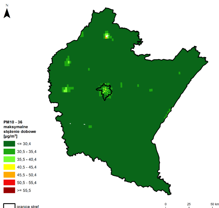
Rysunek 13 Rozkład przestrzenny 36 maksymalnej wartości stężenia 24-godzinnego pyłu PM10 w województwie podkarpackim w 2023 r., będący wynikiem modelowania jakości powietrza dla roku 2021 wykonanego przez IOŚ-PIB [źródło: IOŚ-PIB]
